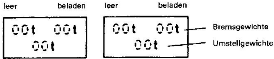
Bild 2 Wagen, die in Bremsstellung „Güterzug“ und „Personenzug“ nur ein Bremsgewicht haben
